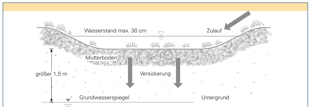
Abb.: Schematischer Aufbau einer Muldenversickerung nach Einstau durch ein Regenergebnis.
